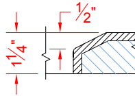
SECTION B-B - SCALE: 3" = 1'-0"
