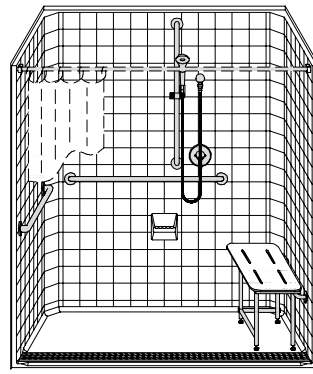
PERSPECTIVE N.T.S.
