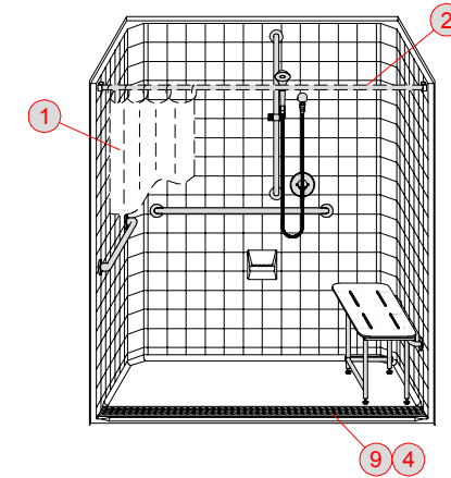
PERSPECTIVE - N.T.S.
